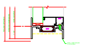
201 SILL 201
