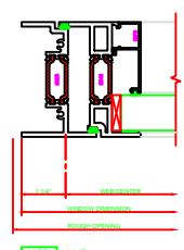
430 JAMB 201
