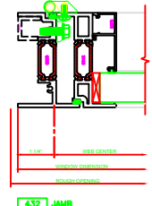
432 JAMB 201
