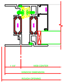
410 JAMB 325 PROJECT III 4-SW. ARM
