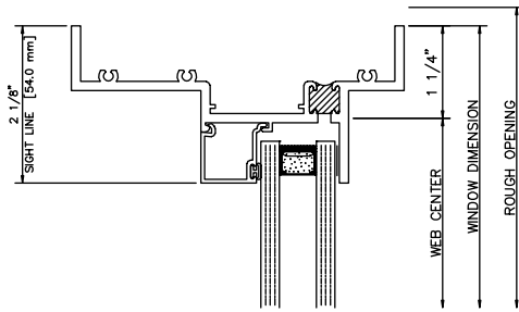
401 RIGHT JAMB
