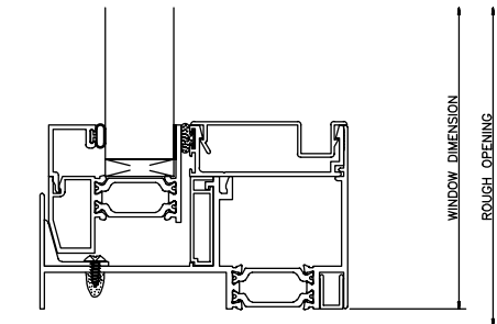
400 LEFT JAMB
