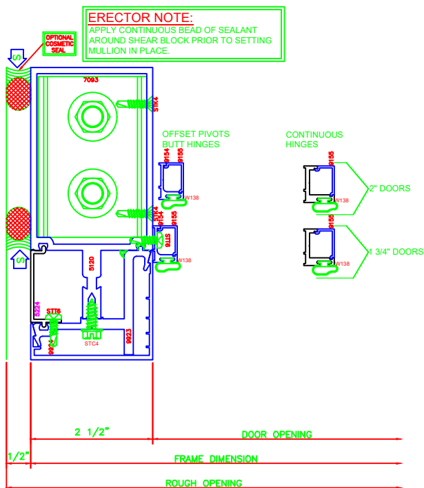
822 O.G. JAMB 5600 6"
