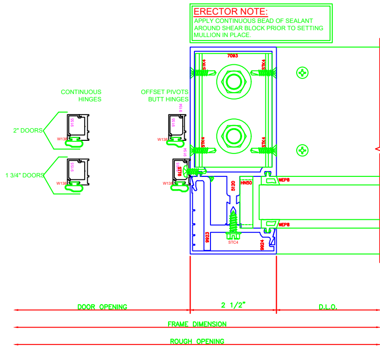
823 O.G. JAMB 5600 6"
