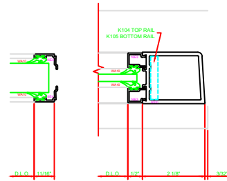
305 STILE S/A D200 FOR OFFSET PIVOT BUTT HINGE
