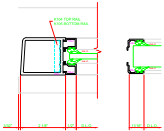
300 STILE S/A D200 FOR OFFSET PIVOT BUTT HINGE
