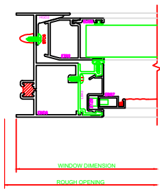
400 JAMB SERIES: 3500
