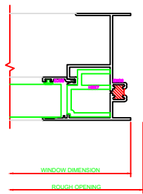
401 JAMB SERIES: 3500
