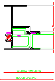
402 JAMB SERIES: 3500
