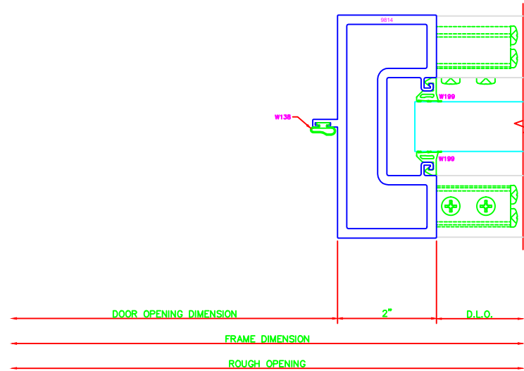
804 DOOR JAMB DURASTILE
