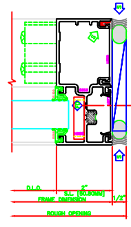
413 RIGHT JAMB S433
