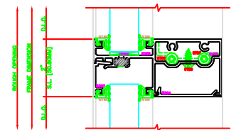
502 O.G. HORZ. S433
