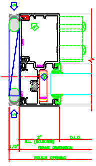
412 LEFT JAMB S433
