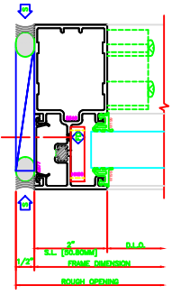
412 LEFT JAMB S433
